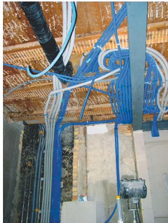
Elektroinstallation
